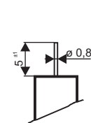
cinovaný drát
