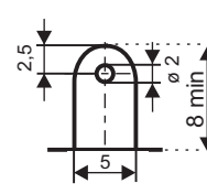
pájecí očka
