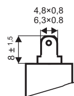
nožové konektory 4,8x0,8 nebo 6,3x0,
